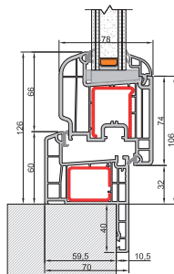
Nodo inferiore Anta maggiorata telaio Z40
