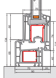
Nodo inferiore Anta maggiorata telaio L
