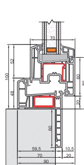
Nodo inferiore Anta squadrata telaio Z60
