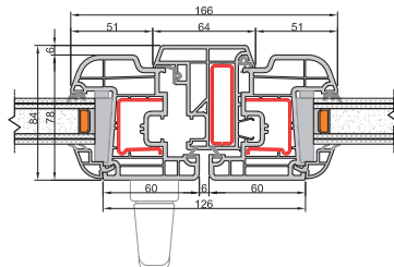
Nodo centrale Anta arrotondata
