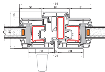
Nodo centrale Anta squadrata
