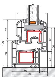
Nodo inferiore Anta arrotondata telaio L
