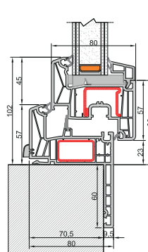
Nodo inferiore Telaio Z60
