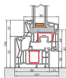
Nodo inferiore Anta slim
