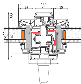
Nodo centrale Anta slim
