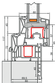
Nodo inferiore Telaio Z40
