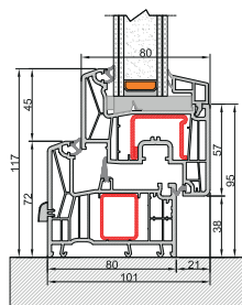
Nodo inferiore Telaio L
