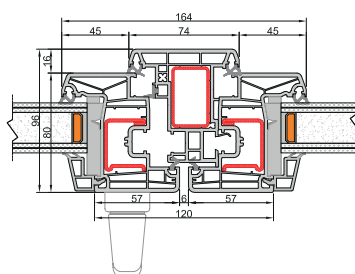
Nodo centrale Anta squadrata
